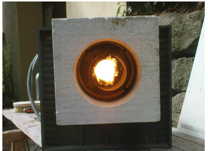
Prolongement du foyer en béton cellulaire
